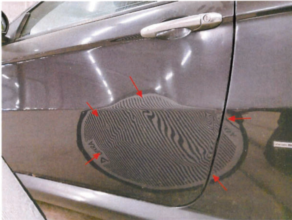
Bild 11 : Tür vorne links, verformt, instandsetzen und lackieren mit Lackaufbau
