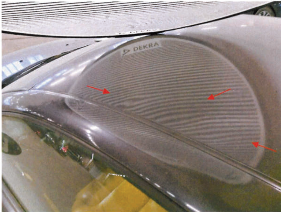
Bild 9 : Dach, mehrfach eingedellt, instandsetzen und lackieren mit Lackaufbau
