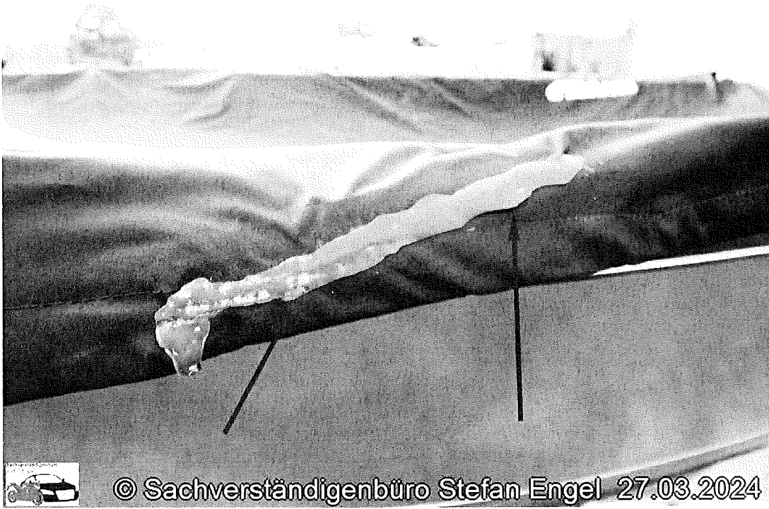
Foto 9: beschädigte Persenning
