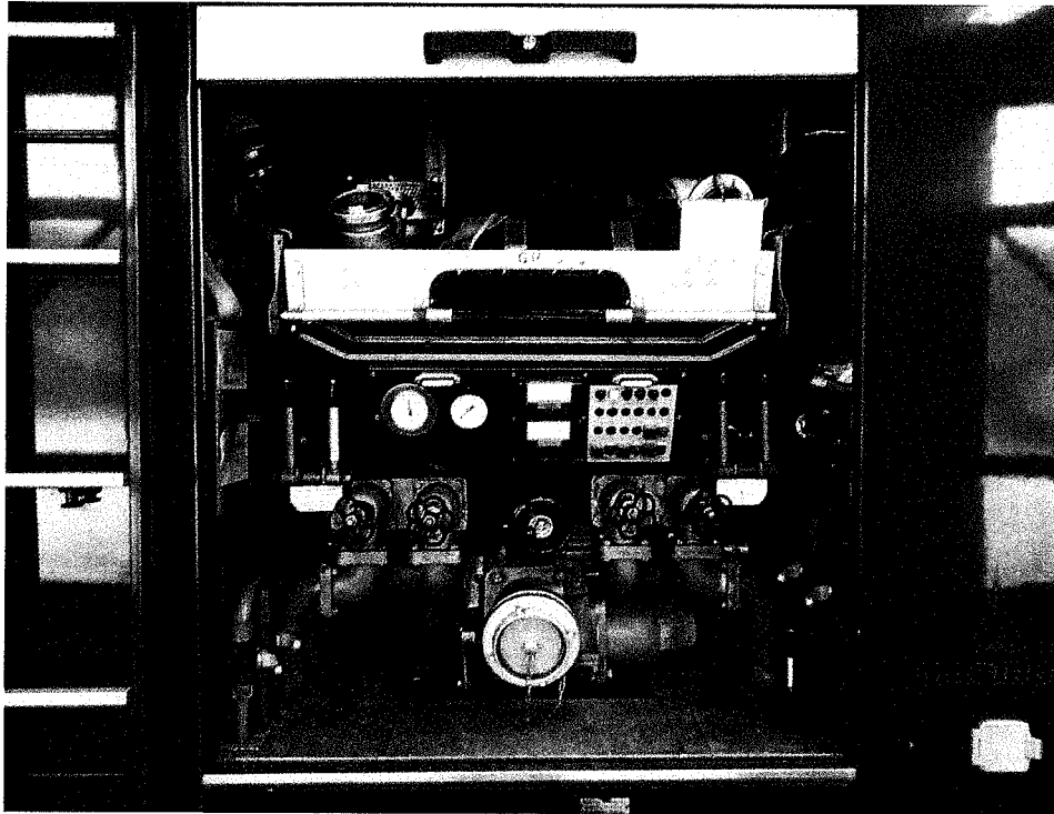
Bild 14 : Aufbauschränke Heck
