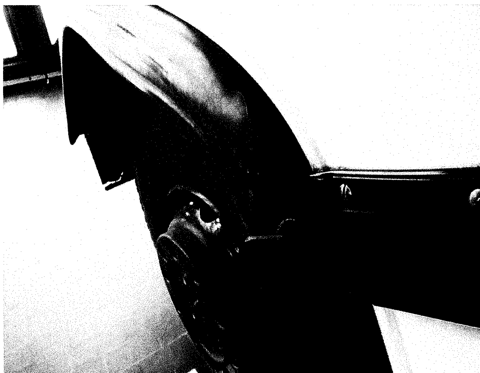
Bild 9 : Radabdeckungen vorne links und rechts gebrochen
